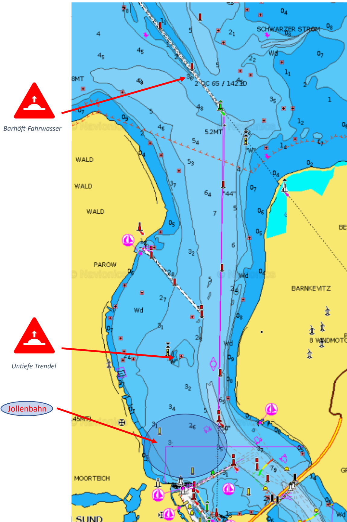
Abbildung 1: Wettfahrtgebiet zwischen Dänholm und Hiddenseefahrwasser (c) navionics
